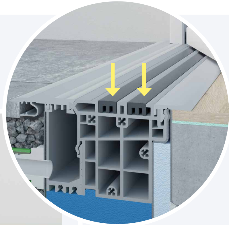
Abbildung: Beide Magnetprofile senken sich beim Öffnen der Tür ab.
