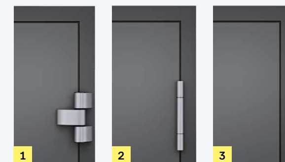
1| Aufschraubband. 2| Rollenband. 3| Verdeckt liegendes Band.
